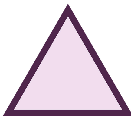
Liksidig triangel
