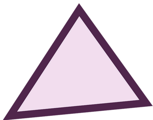
Spetsvinklig triangel
