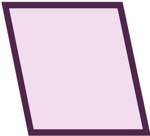
Parallelltrapets
