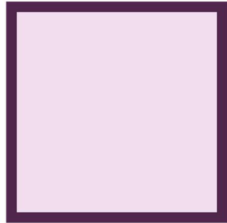
Rektangel
